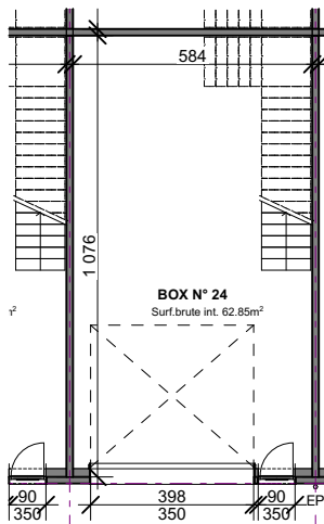
Rez-de-chaussée 1:200
