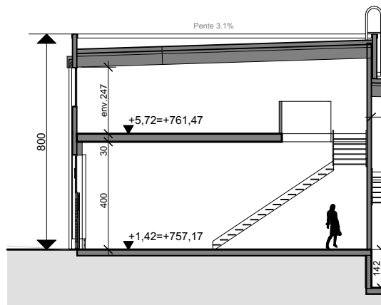
Coupe 1:200
